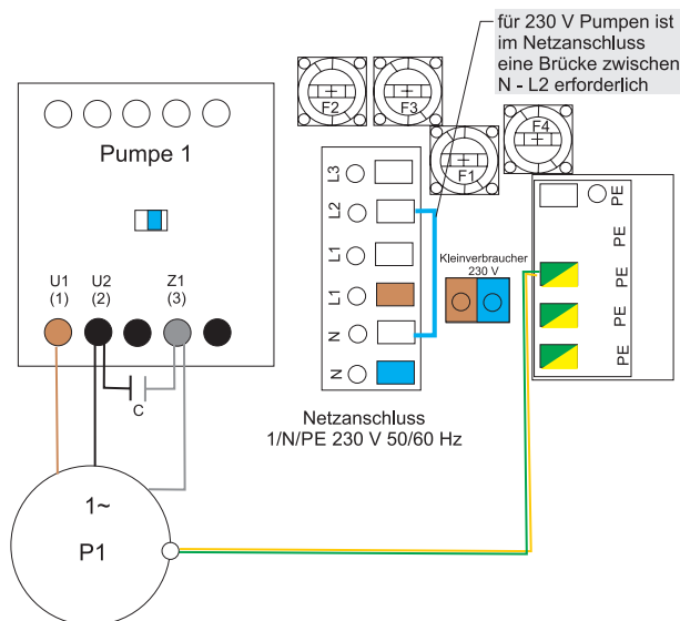
Anschluss 1-Phasen 230 V Wechselstrom-Motor mit externem Kondensator
