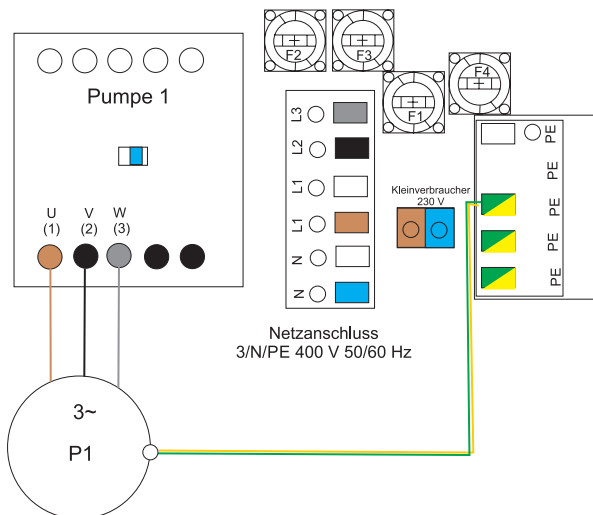
Anschluss 3-Phasen-Motor
