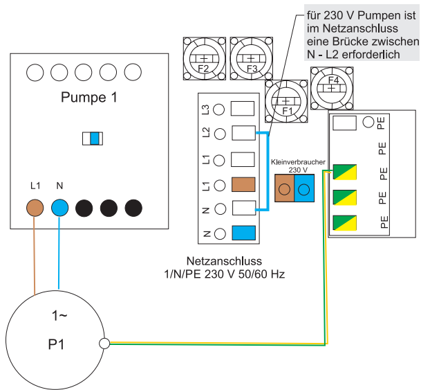
Anschluss 1-Phasen 230 V Wechselstrom-Motor mit internem Kondensator
